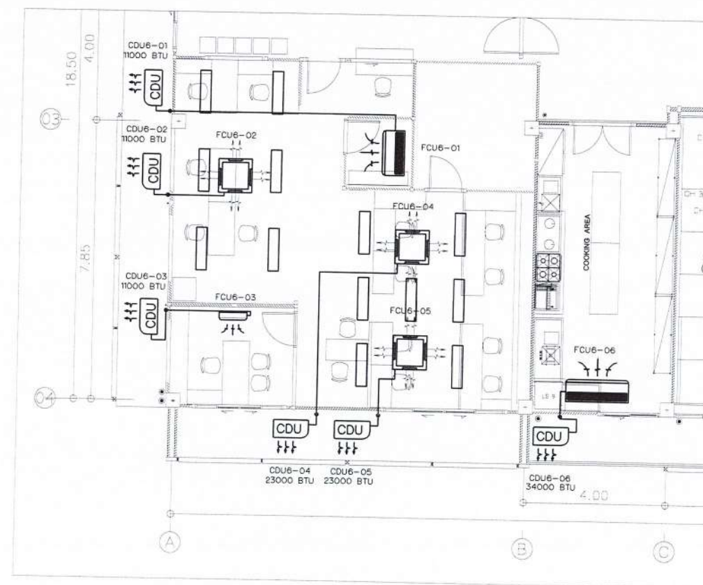
แพลนเครื่องปรับอากาศหมายเลข (FCU6+CDU6)-01 to 06 และแนวท่อน้ำยา ชั้น 6 อาคาร 3
