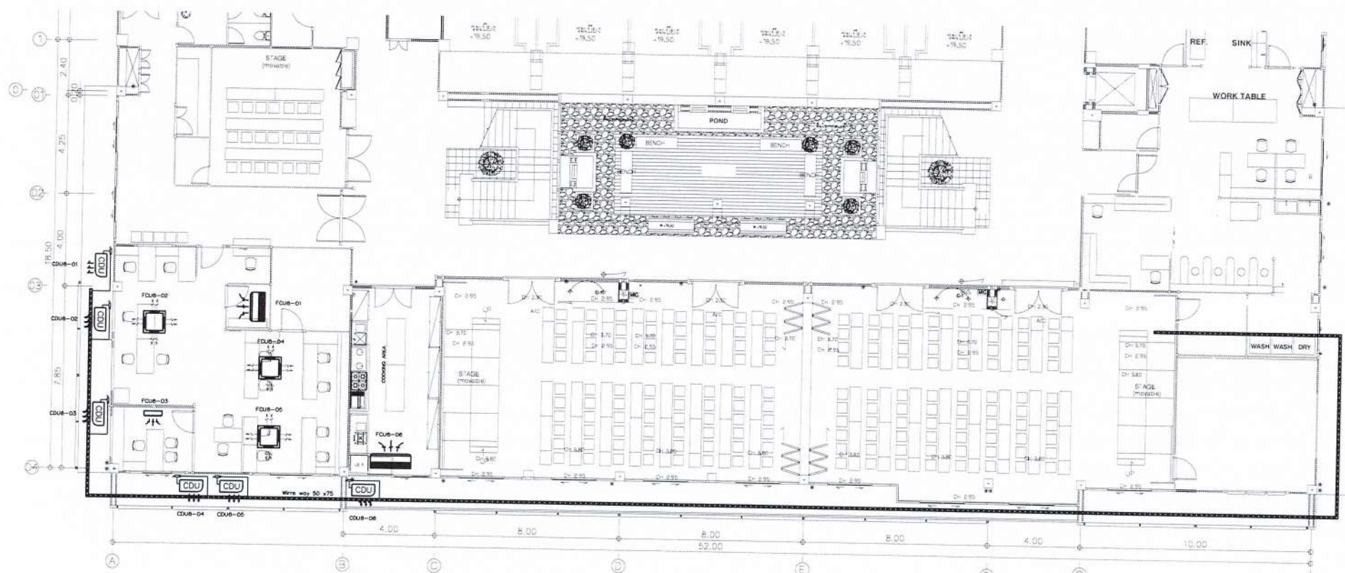
แปลนเครื่องปรับอากาศหมายเลข (FCU6+CDU6) to 06 งานติดตั้ง Safety switch และงานเดินสายไฟฟ้าลงตู้ควบคุม ชั้น 6 อาคาร 3
