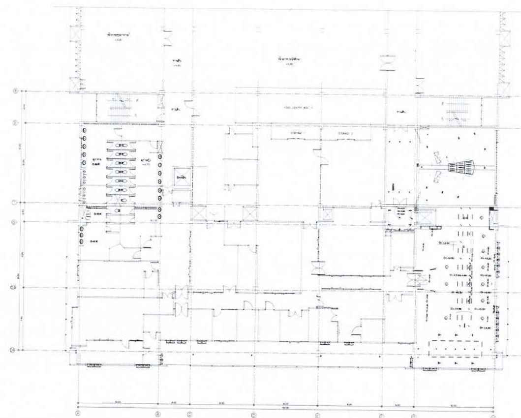
แปลนชุดปรับอากาศหมายเลข (FCU2+CDU2)-01 และงานติดตั้ง Safety switch ชั้น 2 อาคาร 3
