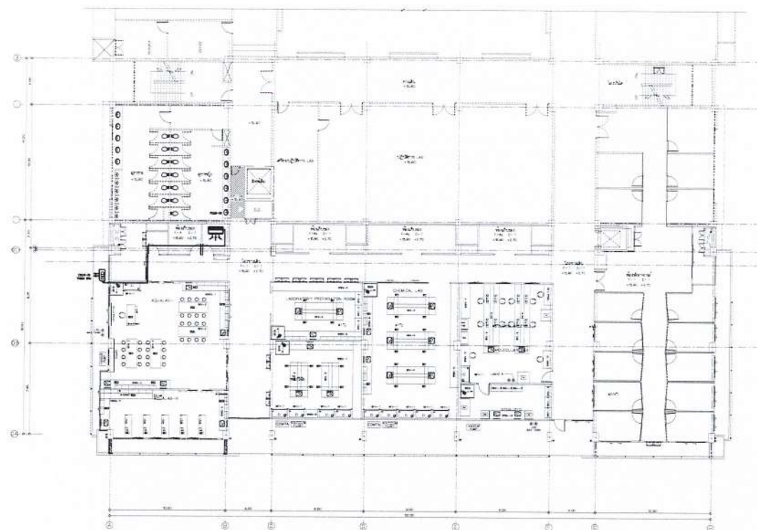
แปลนเครื่องปรับอากาศหมายเลข (FCU5+CDU5)-01 และแนวท่อน้ำยา ชั้น 5 อาคาร 3
