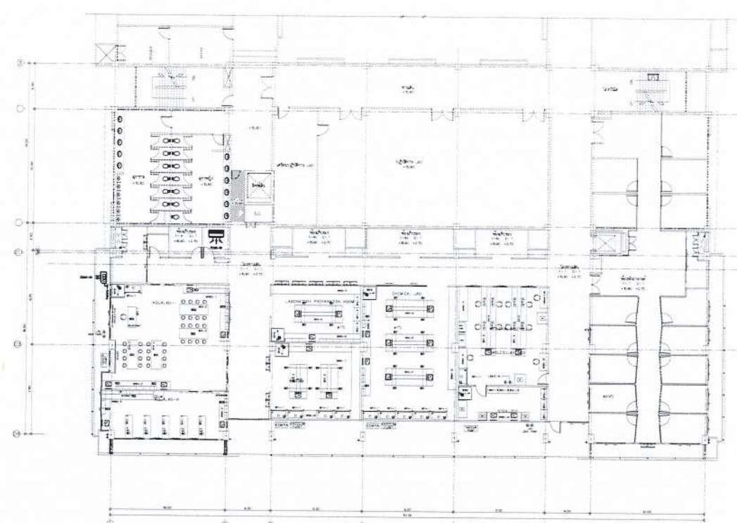
แปลนเครื่องปรับอากาศหมายเลข (FCU5+CDU5)-01 และงานติดตั้ง Safety switch ชั้น 5 อาคาร 3
