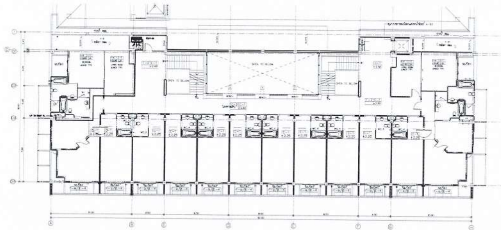
แปลนเครื่องส่งลมเย็นหมายเลข FCU7-01 และแนวท่อน้ำยา ชั้น 7 อาคาร 3
