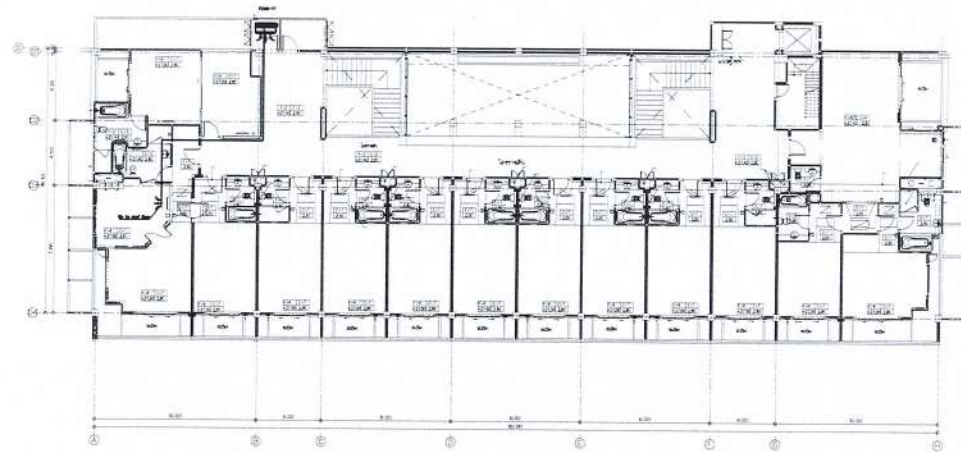
แปลนเครื่องส่งลมเย็นหมายเลข FCU8-01 และแนวท่อน้ำยา ชั้น 8 อาคาร 3
