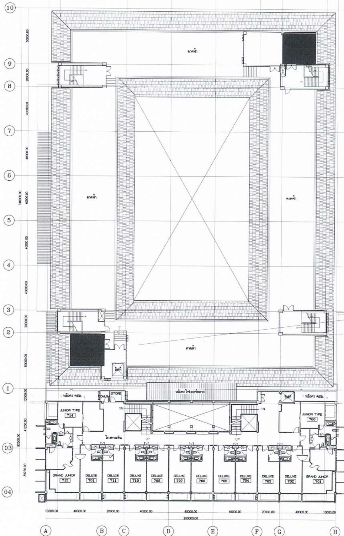
แปลนพื้นที่ชั้นดาดฟ้า อาคาร 1
