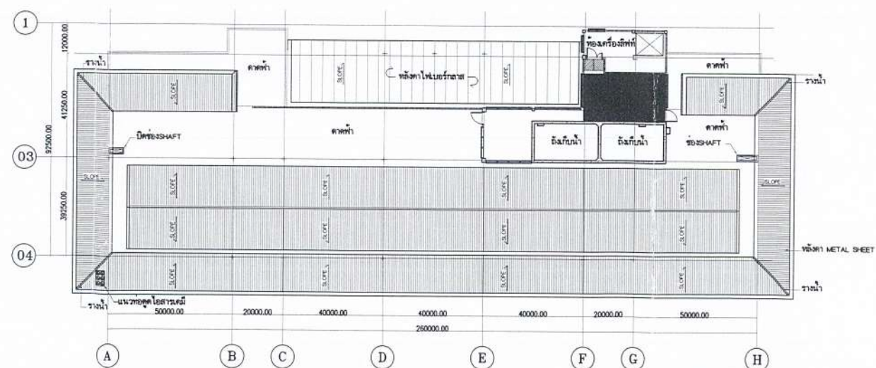
แปลนพื้นที่ชั้นดาดฟ้า อาคาร 3
