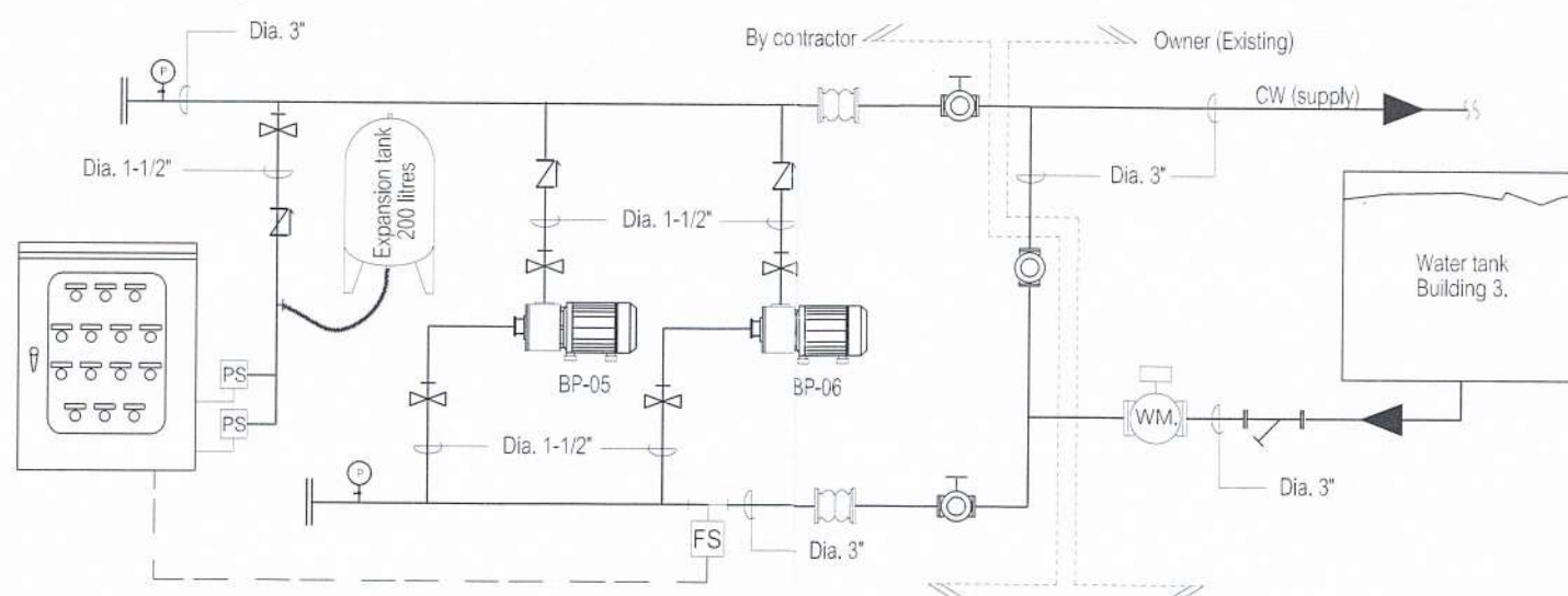
Diagram Booster pump หมายเลข BP-05 และ 06
