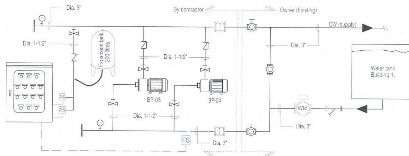
Diagram Booster pump หมายเลข BP-03 และ 04
