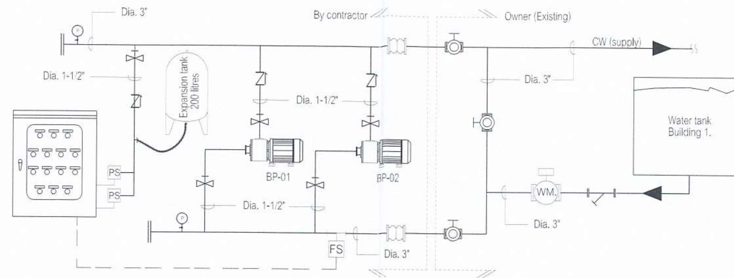
Diagram Booster pump หมายเลข BP-01 และ 02
