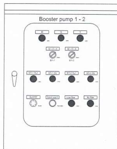
ภาพขยายตู้ควบคุมเครื่องสูบน้ำรักษาแรงดัน
